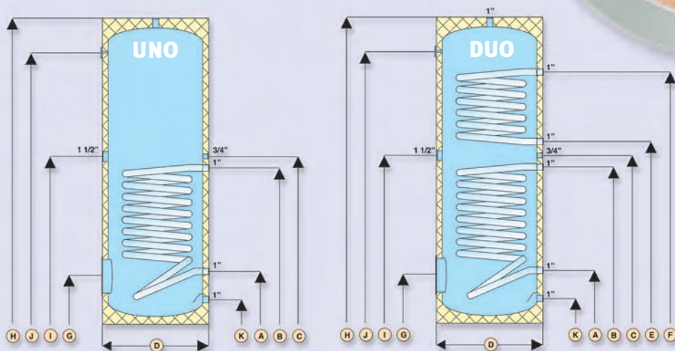
Abmessungen (mm)
